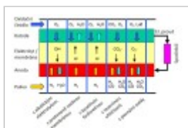
Obrázek 4 Souhrn principů různých typů palivových článků
